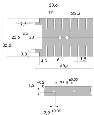
FORATURA SUGGERITA SU PCB RECOMMENDED PCB HOLES LAYOUT
